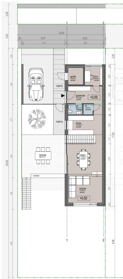
Erdgeschoß
